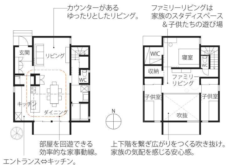
1階平面図
